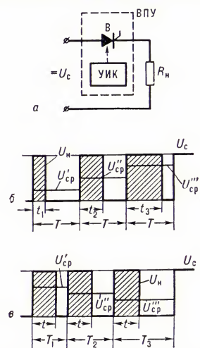
Рис. 3. Схема полупроводникового вентильного регулятора постоянного тока (а) и диаграммы его напряжений (б, в): T — интервалы следования управляющих импульсов (на отпираание вентиля); t — продолжительность открытого состояния вентиля; остальные обозначения те же, что и на рис. 1.
